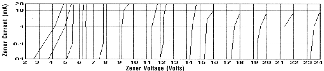
Zener Current vs. Zener Voltage
